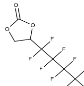
3,3,4,4,5,5,6,6,6-Nonafluorohexyl-1-ene carbonate
