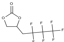
4-(2,2,3,3,4,4,4-Heptafluorobutyl)-1,3-dioxolan-2-one
