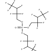
Tris(2,2,3,3,4,4,4-hexafluorobutyl)phosphate
