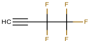
3,3,4,4,4-Pentafluoro-1-butyne 1500-3-06 [7096-51-7]
