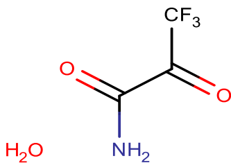
Trifluoropyruvamide monohydrate 4148-3-22 [1210756-85-6]
