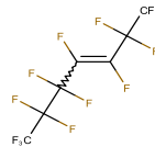
Perfluorohept-3-ene
