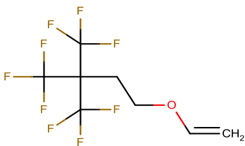
3,3-Bis(trifluoromethyl)-4,4,4-trifluorobutyl vinyl ether 2307-3-0C []
