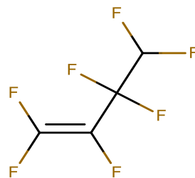
1,1,2,3,3,4,4-Heptafluorobut-1-ene 1300-3-50 [680-54-6]
